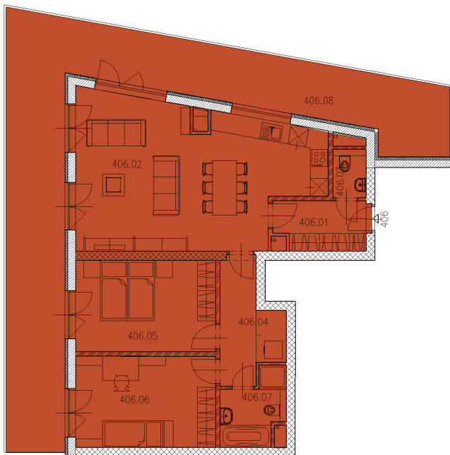
1 půdorys bytu
